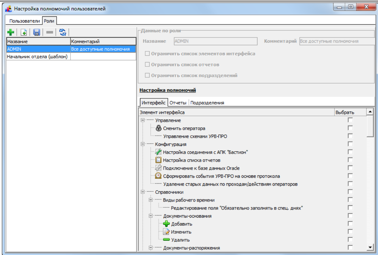
Рис. 9. Настройка ролей
